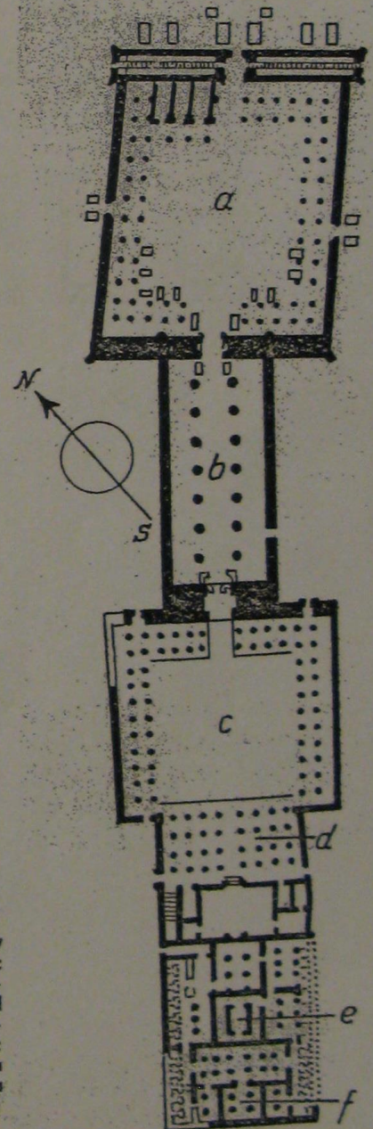
Plan świątyni Amona w Luksorze: a – dziedziniec Ramzesa II, b – kolumnada Amenhotepa III uzurpowana przez Ho-remheba, c – dziedziniec Amenhotepa III, d – sala hypostylowa, e – sala na barcę, f – kaplica. XVIII dynastia
